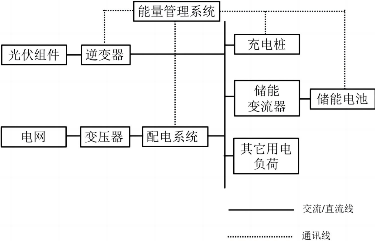
图A.1 光储充一体化电站架构
